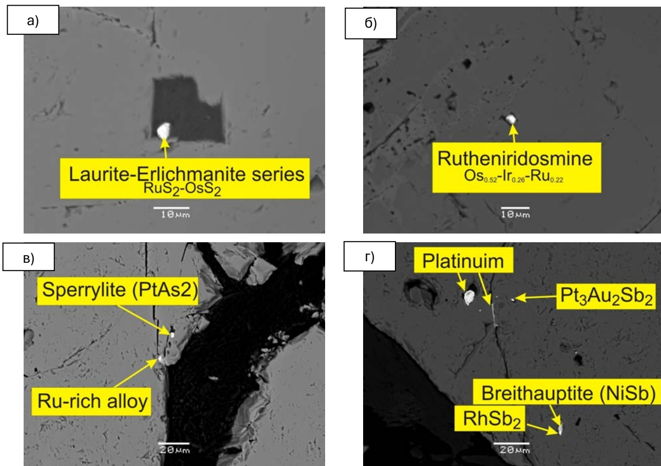
Рис. 76. Обратное рассеянные изображения в отраженных электронах (BSE) сплавы и минералы ЭПГ в исследуемом хромите. Составлено автором.
