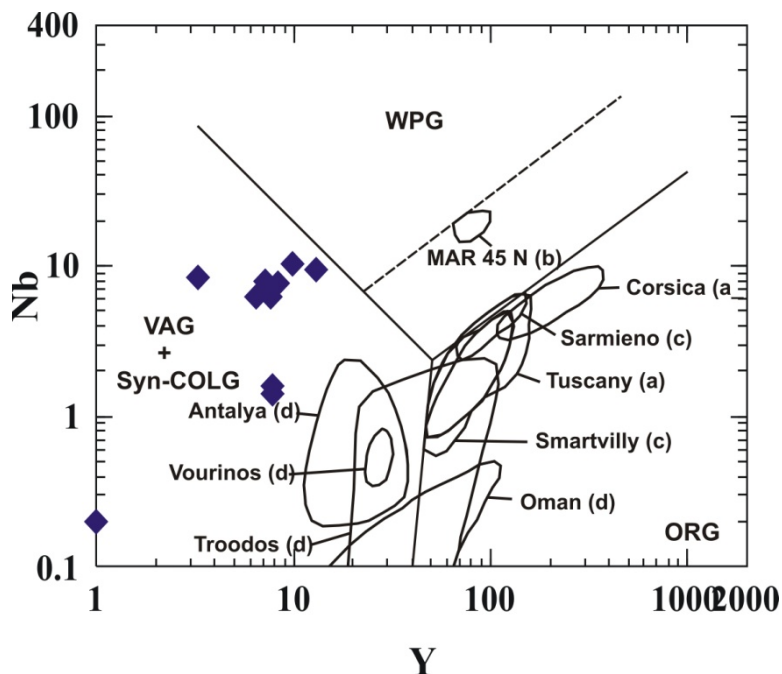
Рис. 56. Дискриминационная диаграмма Nb-Y для анализируемого плагиигранита. Поля: внутриплитные граниты (WPG) + граниты океанических хребтов (ORG) и граниты вулканической дуги (VAG) + синколлизийные граниты (syn-COLG) указаны по Pearce et al. (1984a). Анализируемые плагииграниты залегают в гранитах вулканической дуги и в коллизийных гранитах. Составлено автором.
