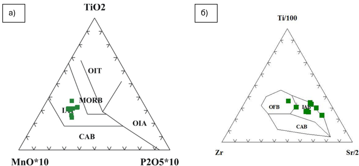
Рис. 66. Геохимическая диаграмма и диаграмма тектонической обстановки массива Кала Эн Нахаль: а) TiO_2 - MnO * 10 - P_2O_5 * 10 . Поля: MORB = базальт срединно-океанического хребта; OIT = толеиты океанических островов; OIA = андезиты океанических островов; CAB = известково-щелочные базальты; IAT = островодужные толеиты по Mullen (1983); б) диаграмма Ti / 100 -Zr-Sr / 2 по Pearce and Cann (1973). OFB: базальты океанического дна (MORB); IAB: островодужные базальты; CAB: известково-щелочной базальт. Составлено автором.
