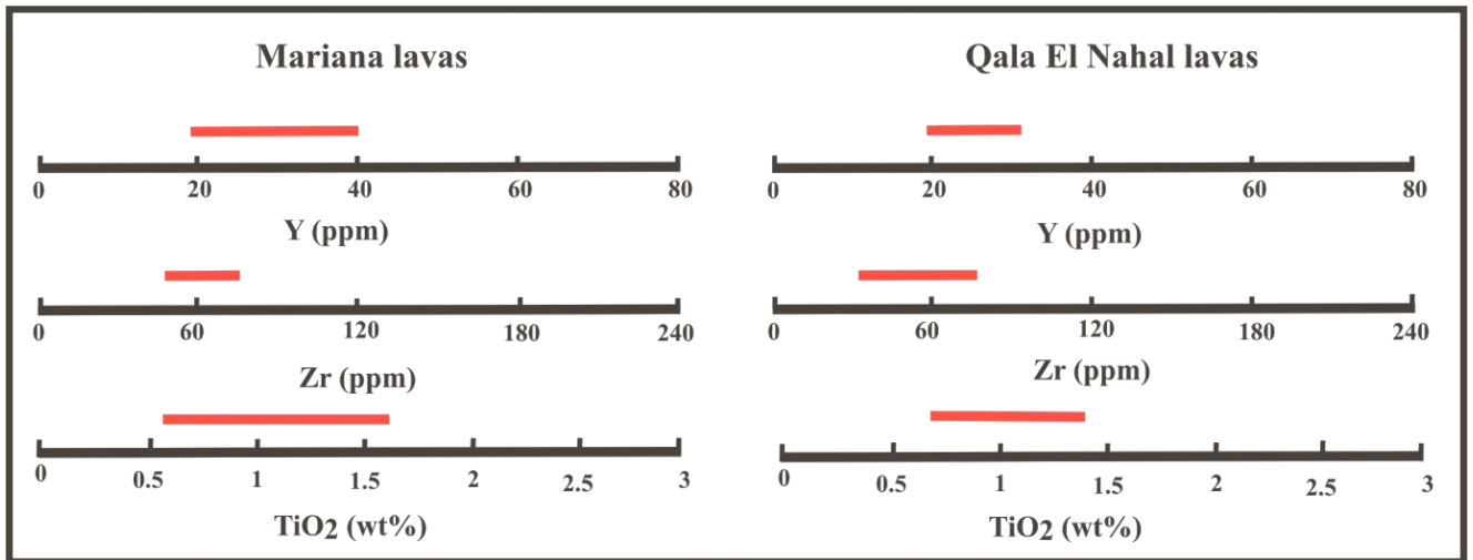
Рис. 70. Дискриминационная диаграмма \text{TiO}_2 (мас. %), Zr (ppm) и Y (ppm) между лавами Кала Эн Нахаль и лавами преддуги Марианских островов (Марианской преддуги). Составлено автором.
