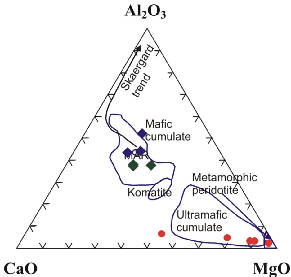
Рис. 46. Диаграмма соотношений CaO-Al_2O_3-MgO анализируемых габброидов. Анализируемые образцы попадают в поле основных кумулятивных пород. Поля по Coleman (1977). Составлено автором.
