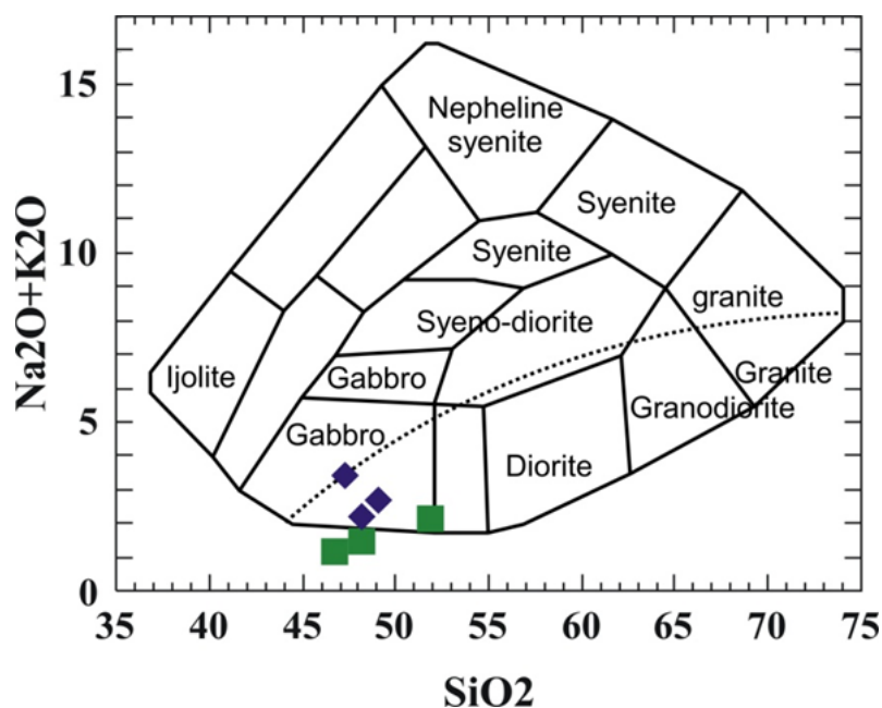
Рис. 47. Диаграммы классификации основной кумулятивной породы изученного офиолита. a-TAS-диаграмма (диаграмма сумма щелочей — кремнезема (TAS) (Cox et al. 1979). Составлено автором.
