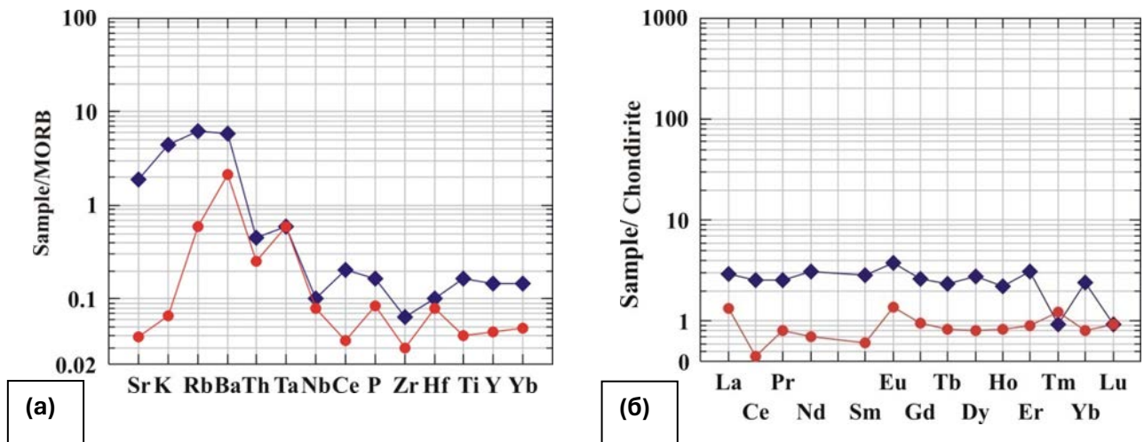
Рис.49. а) MORB-нормированный микроэлемент для исследуемого кумулята. Нормированные значения приведены в работе Veivins и др. (1984) ; б) Нормализованные по хондриту РЗЭ для изученных кумулятов. Нормированные значения – это значения Бойнтонна ( Boynnton, 1984 ).
